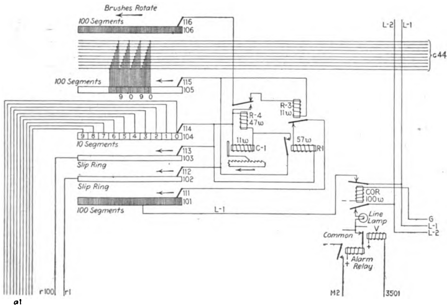
FIG. 139.—Decimal indicator circuit.
