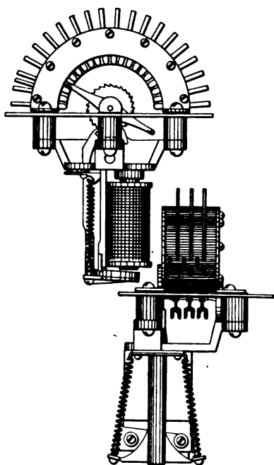
FIG. 190.—Rotary switch.
