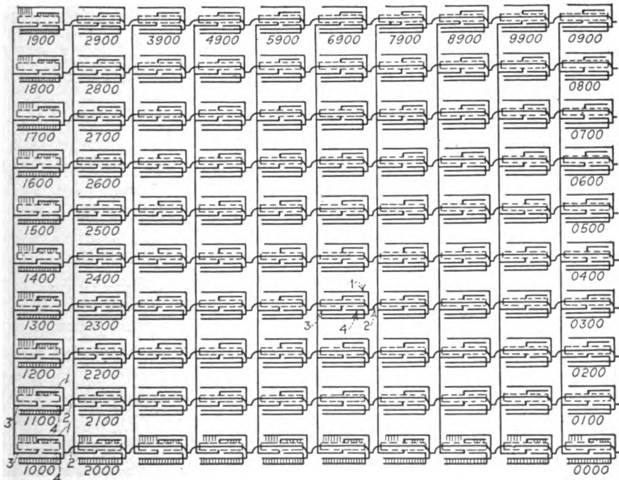
FIG. 7.—Floor plan, Keith trunking (U. S. Pat. 831,876 floor plan, Fig. 1).
