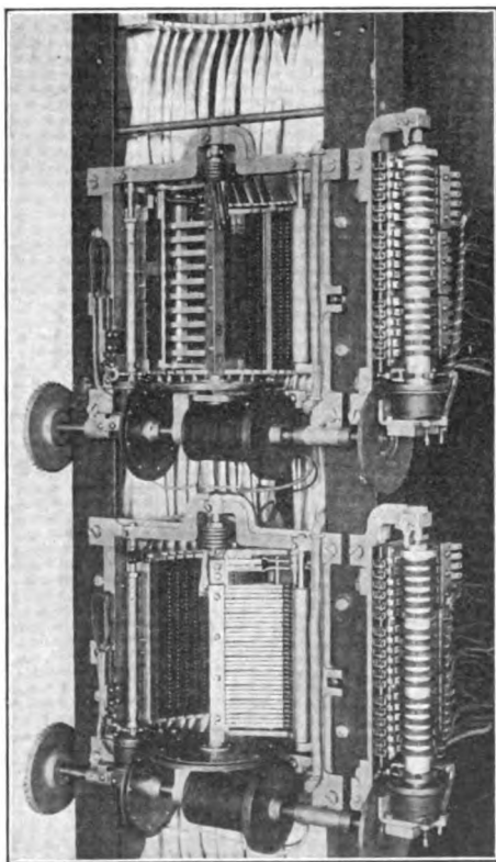
FIG. 200.—Selector.
