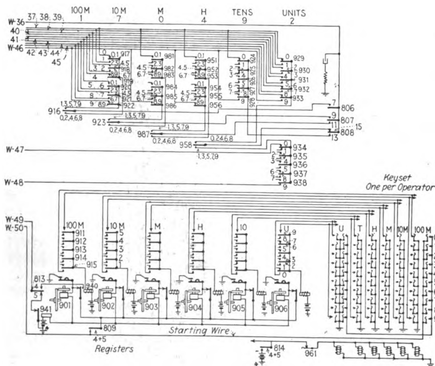
FIG. 218.—Register circuit.
