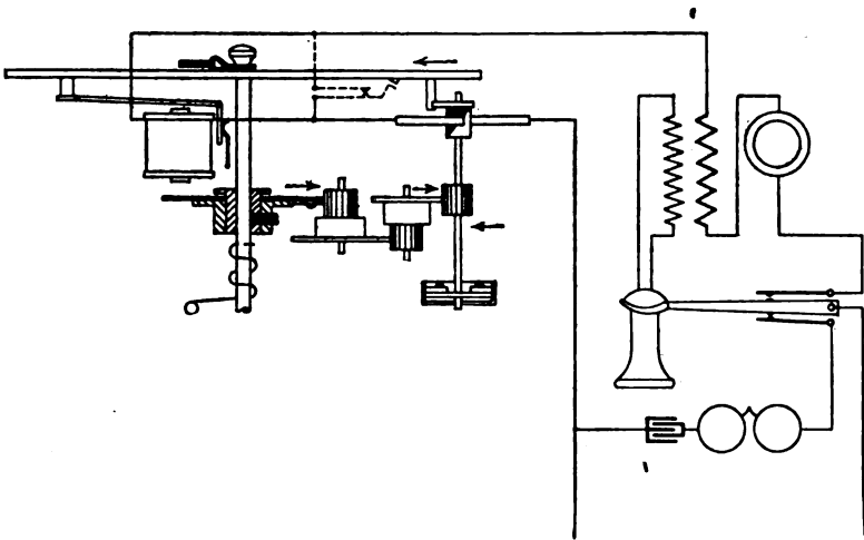
FIG. 93.—Telephone circuit.
