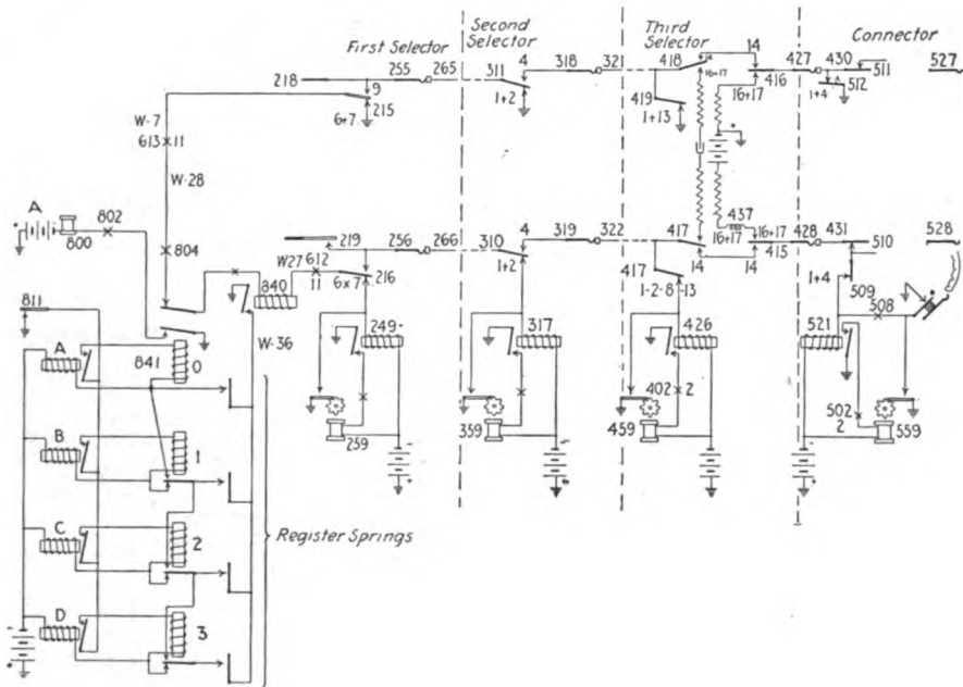
FIG. 224.—Fundamental circuit.
