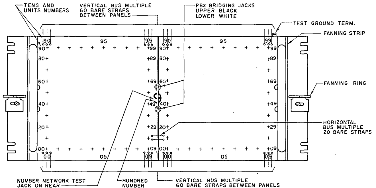
Fig. 5—Number Network Panel (313A)—200 Numbers
