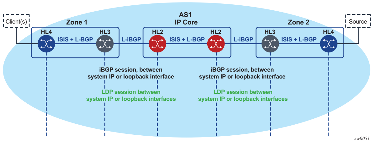
Figure 80 ABR and iBGP
