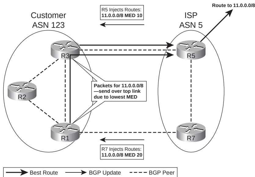
Figure 13-11 Typical Use of MED
